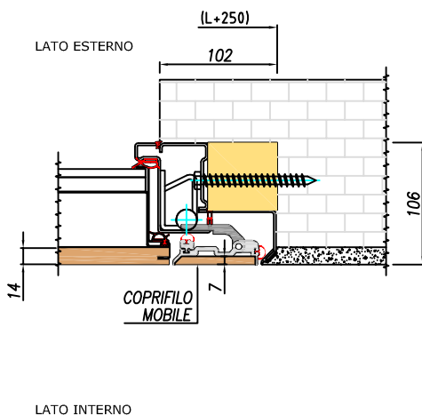
SEZIONE TRASVERSALE - lato cerniere
