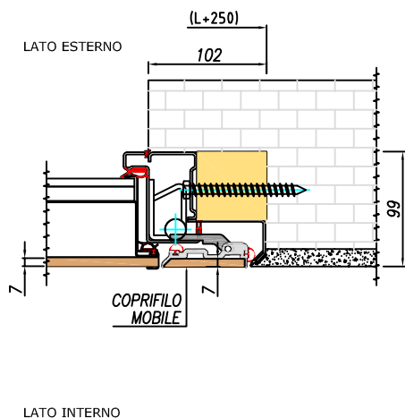
SEZIONE TRASVERSALE - lato cerniere
