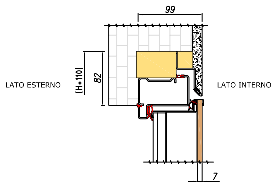
SEZIONE TRASVERSALE - lato cerniere
