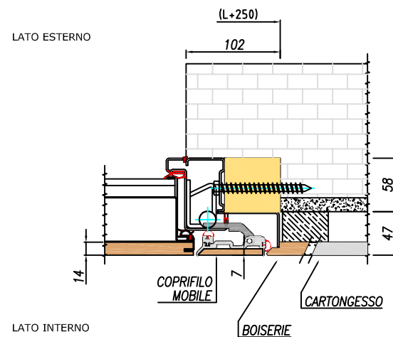
SEZIONE TRASVERSALE - lato cerniere
