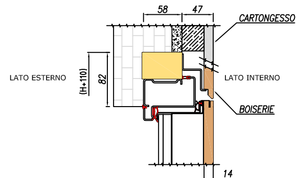
SEZIONE LONGITUDINALE
