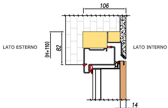
SEZIONE LONGITUDINALE
